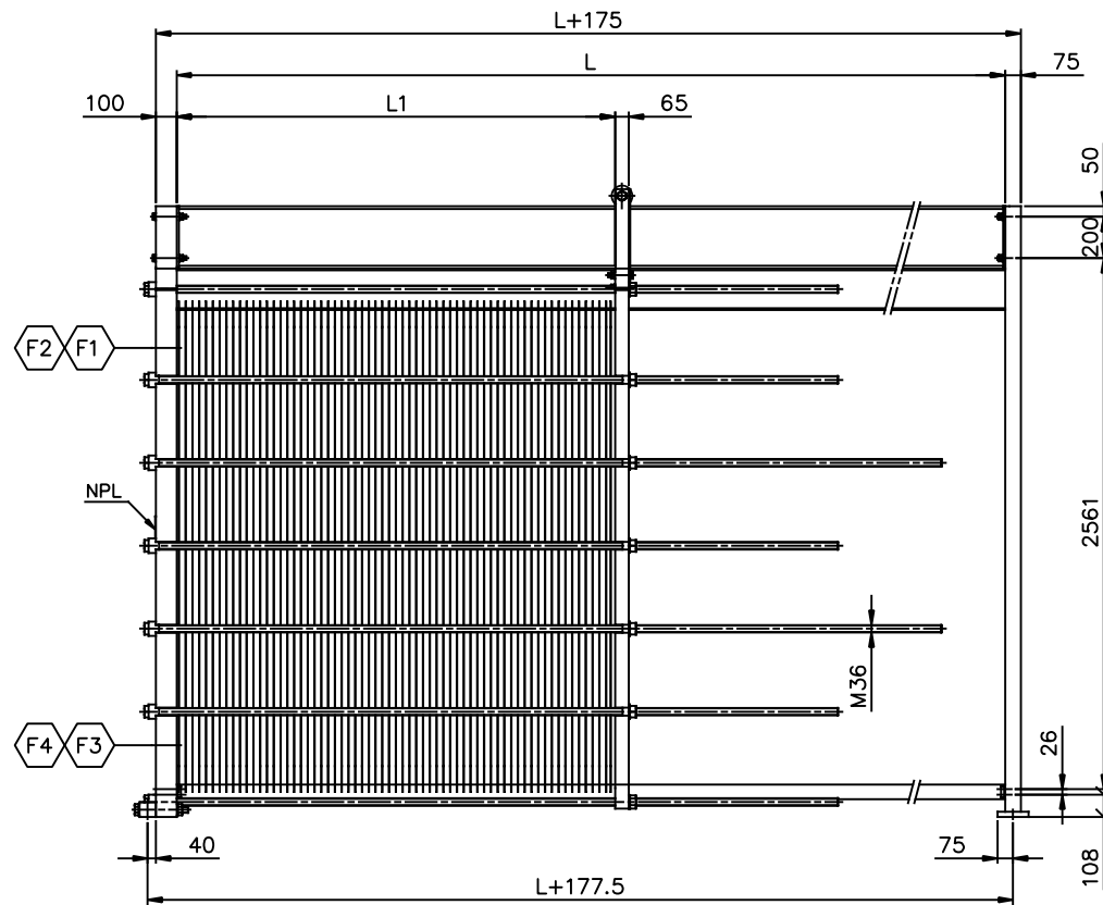
ELEVATION SCALE: 1/20
