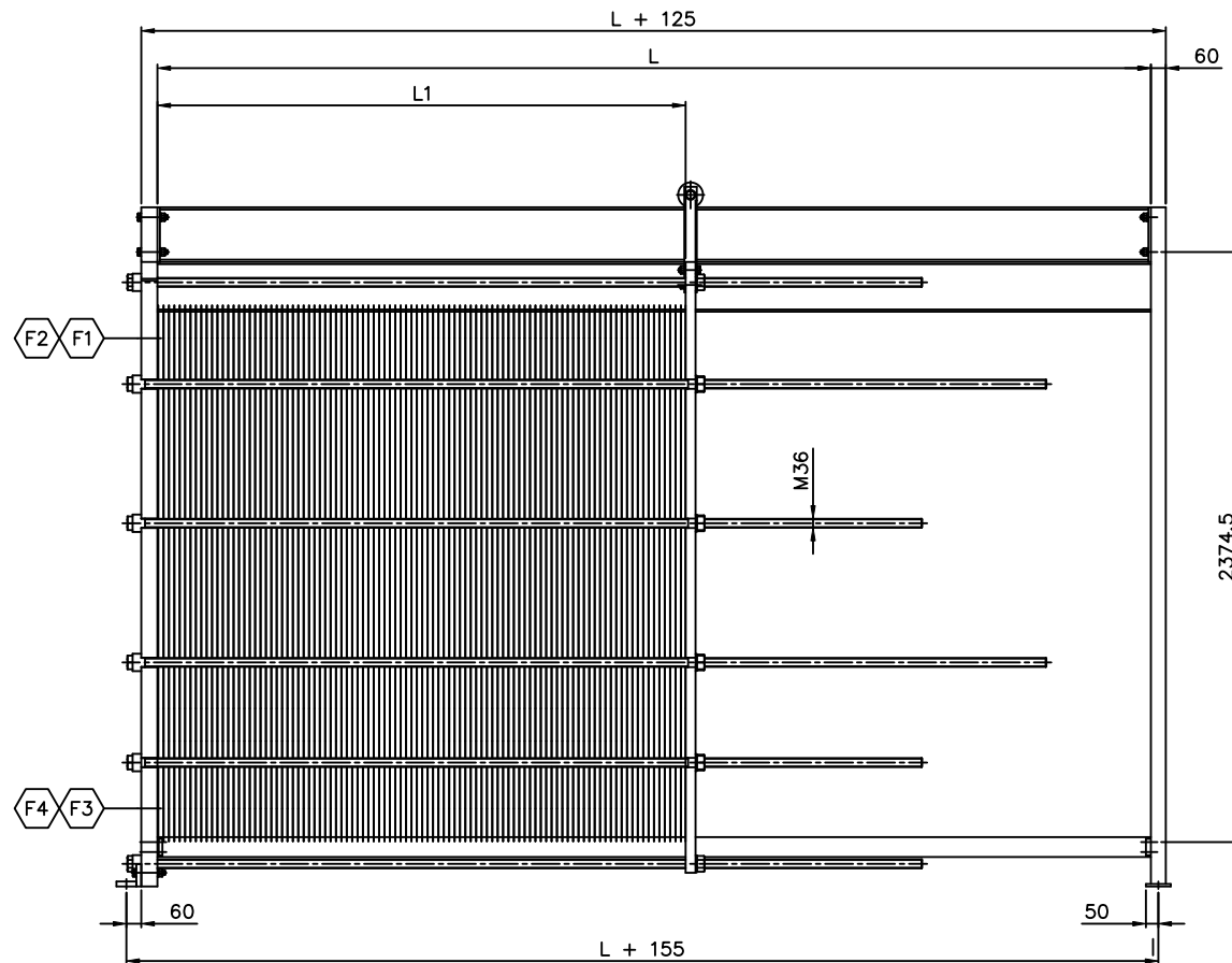
ELEVATION SCALE: 1/15
