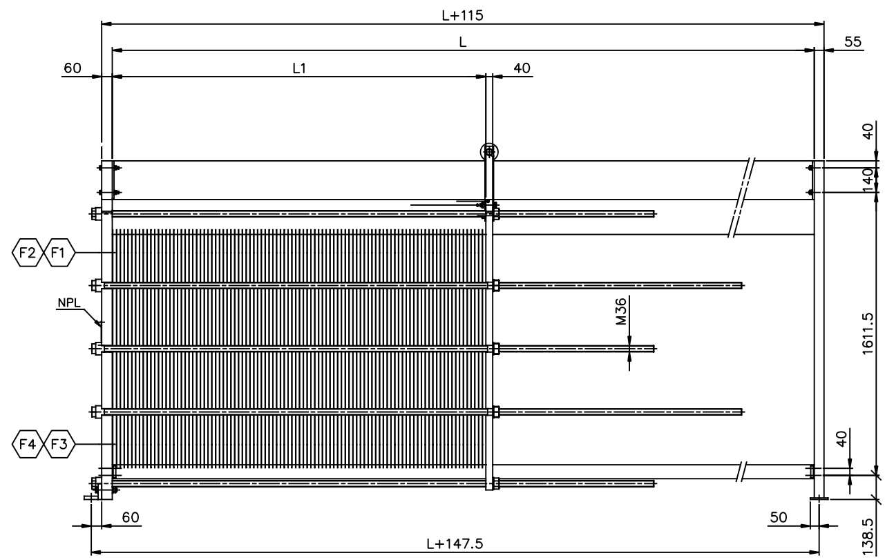
ELEVATION SCALE: 1/15
