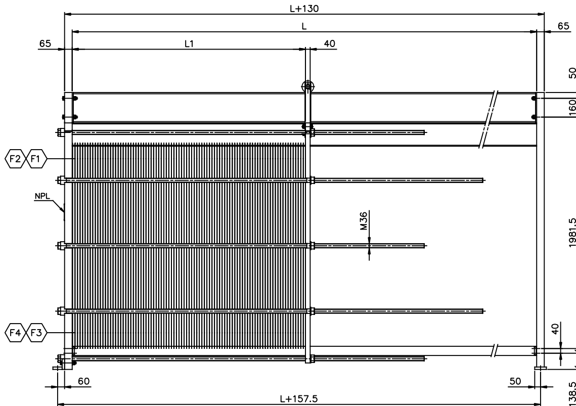
ELEVATION SCALE: 1/15
