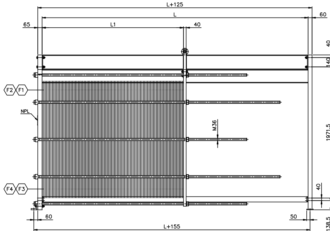
ELEVATION SCALE: 1/15
