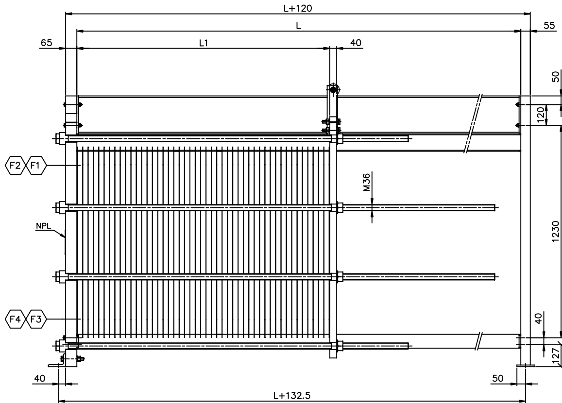
ELEVATION SCALE: 1/10
