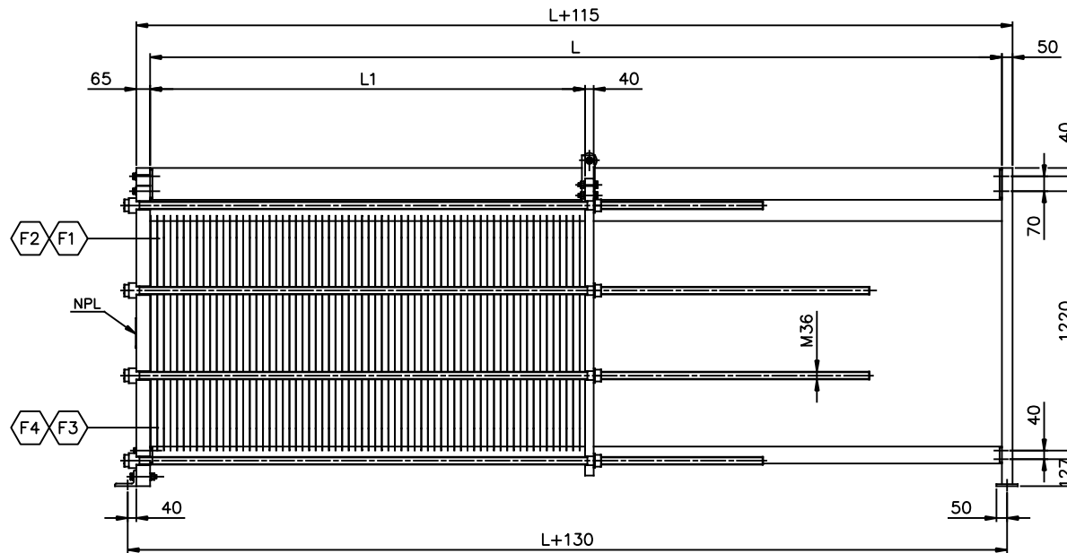
ELEVATION SCALE: 1/15
