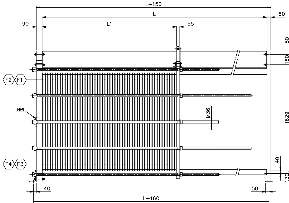
ELEVATION SCALE: 1/15
