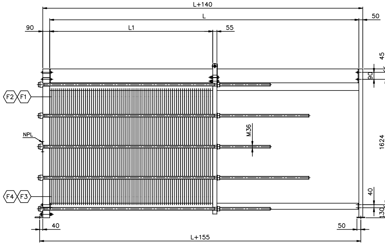
ELEVATION SCALE: 1/15
