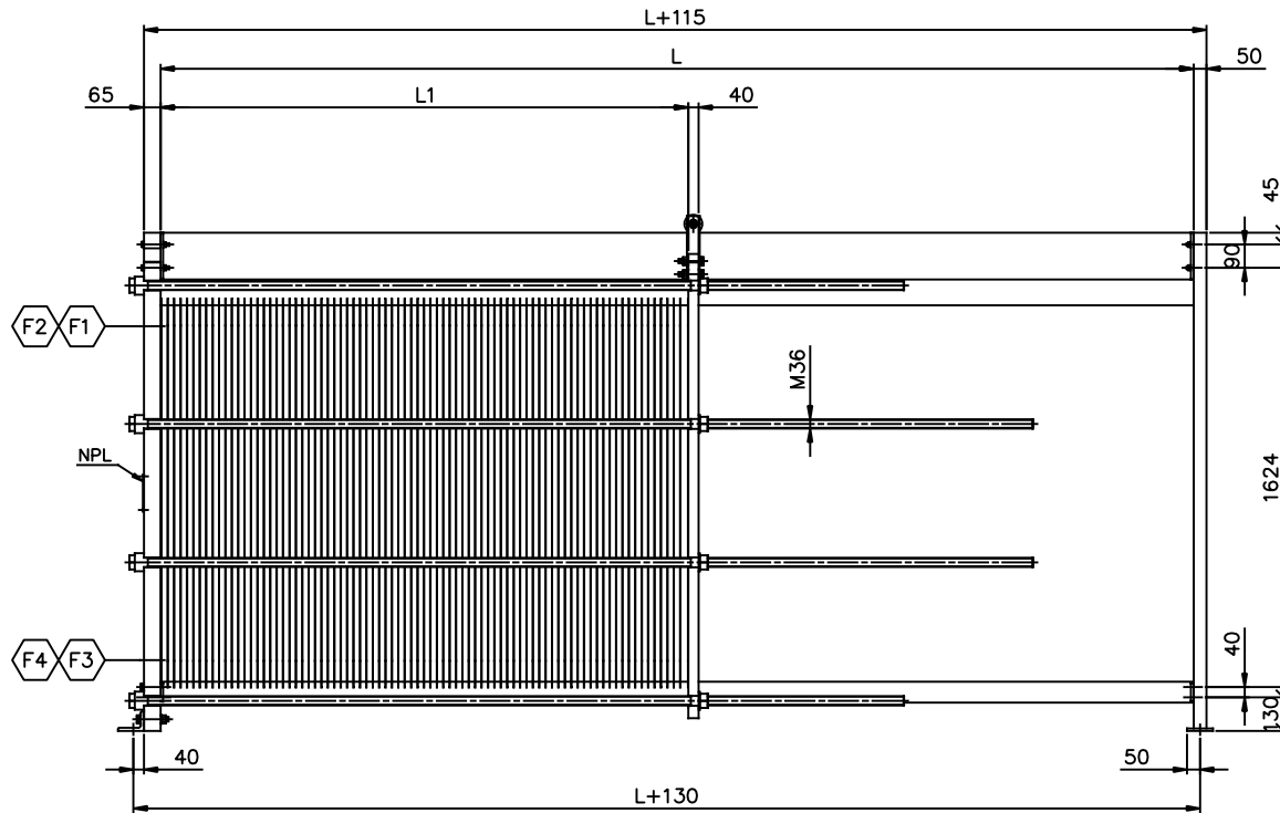
ELEVATION SCALE: 1/15
