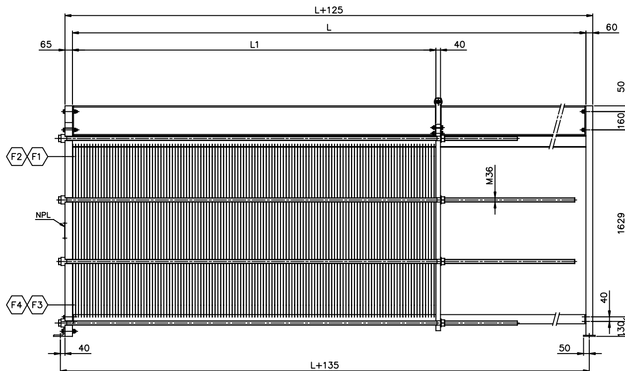
ELEVATION SCALE: 1/15
