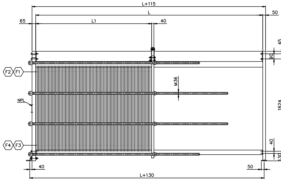
ELEVATION SCALE: 1/15
