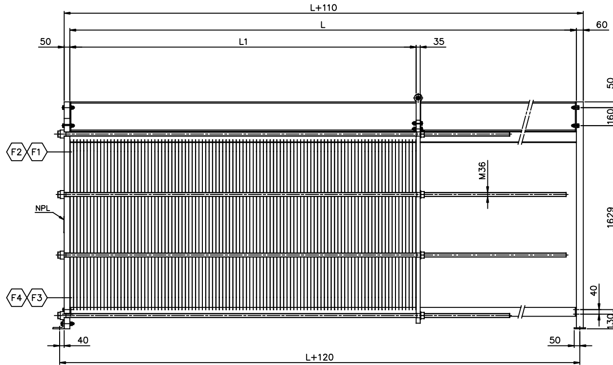
ELEVATION SCALE: 1/15
