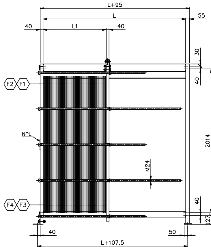
ELEVATION SCALE: 1/15
