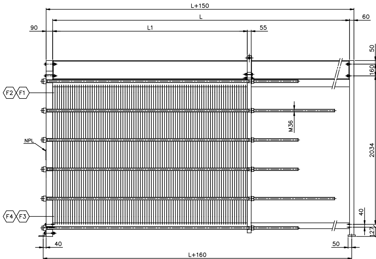
ELEVATION SCALE: 1/15
