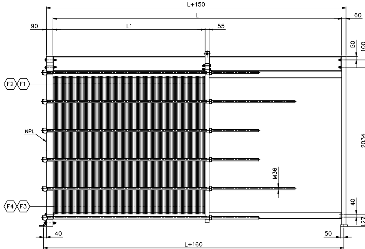
ELEVATION SCALE: 1/15
