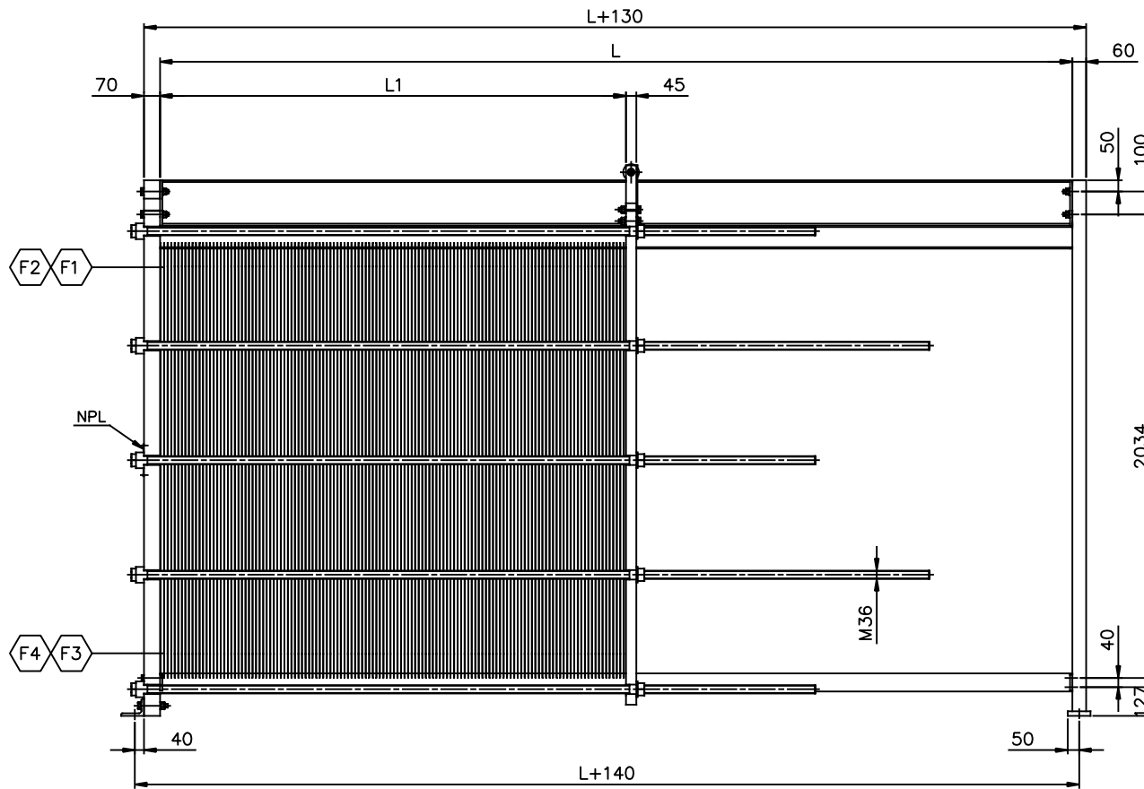
ELEVATION SCALE: 1/15
