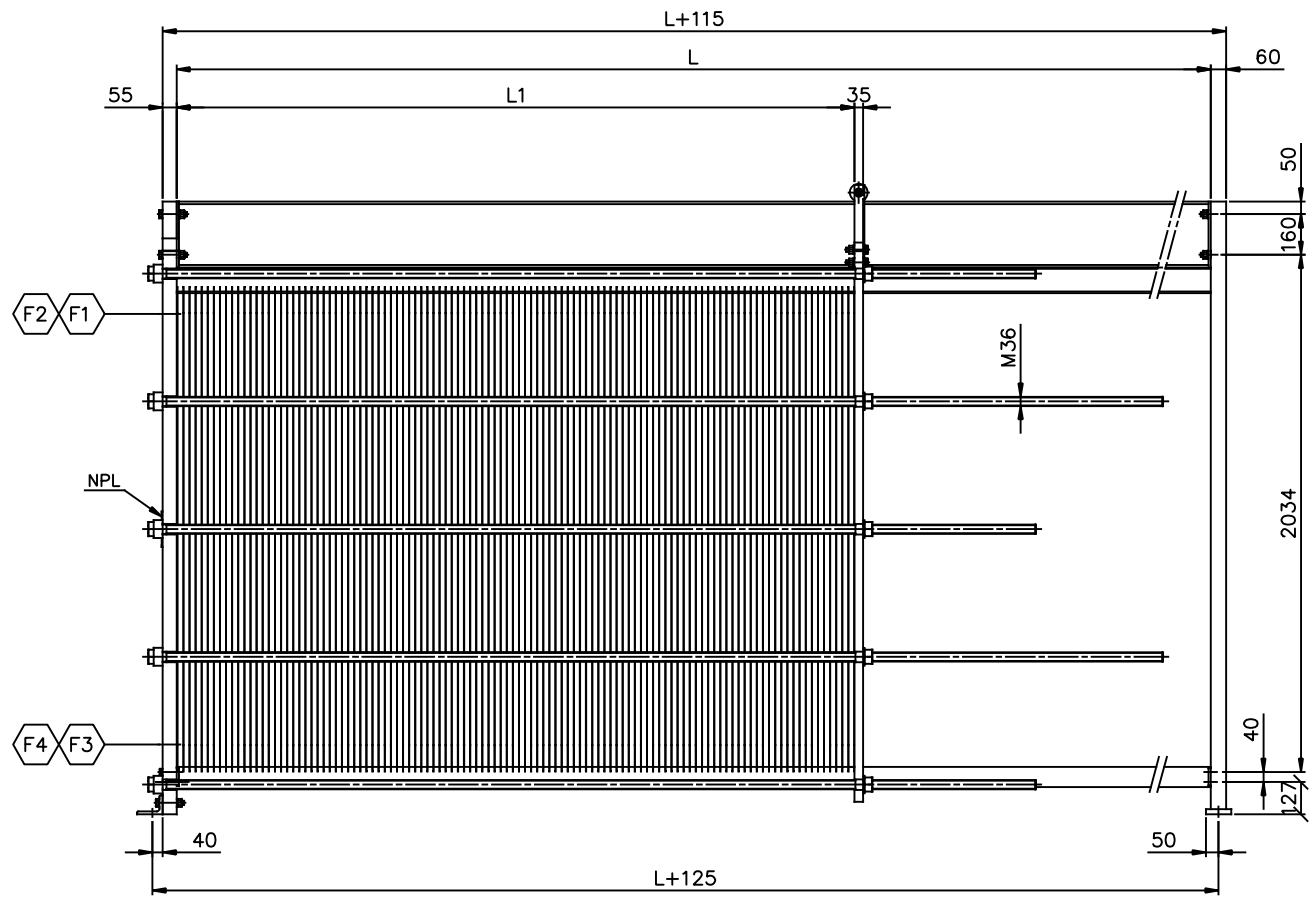
ELEVATION SCALE: 1/15
