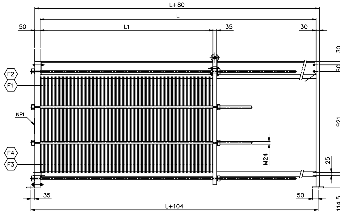
ELEVATION SCALE: 1/10
