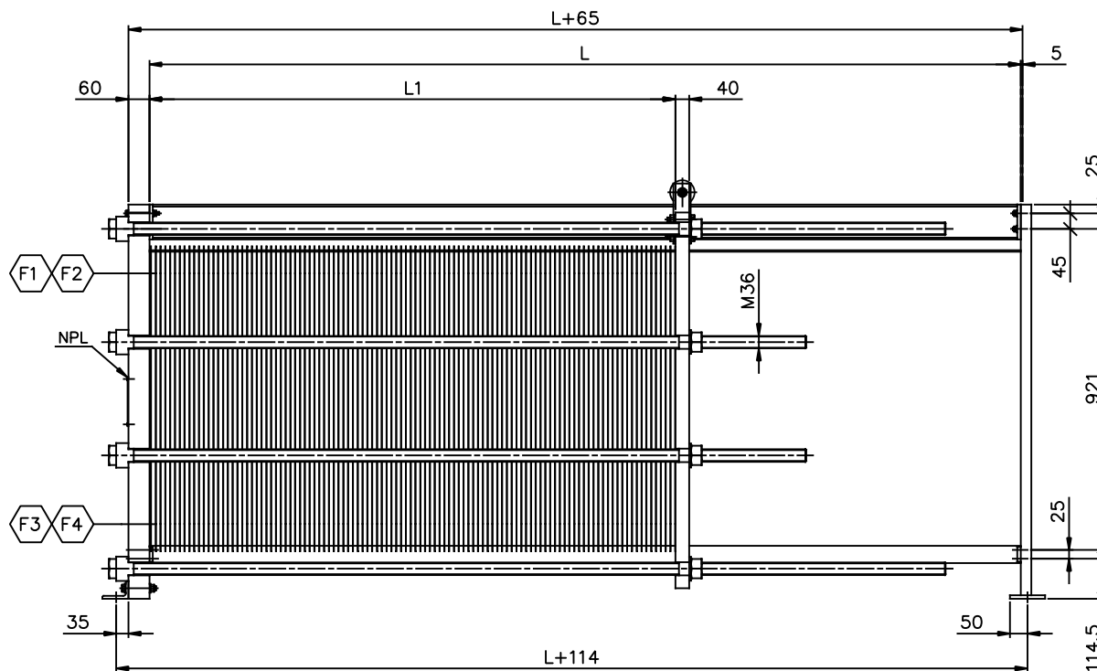
ELEVATION SCALE: 1/10
