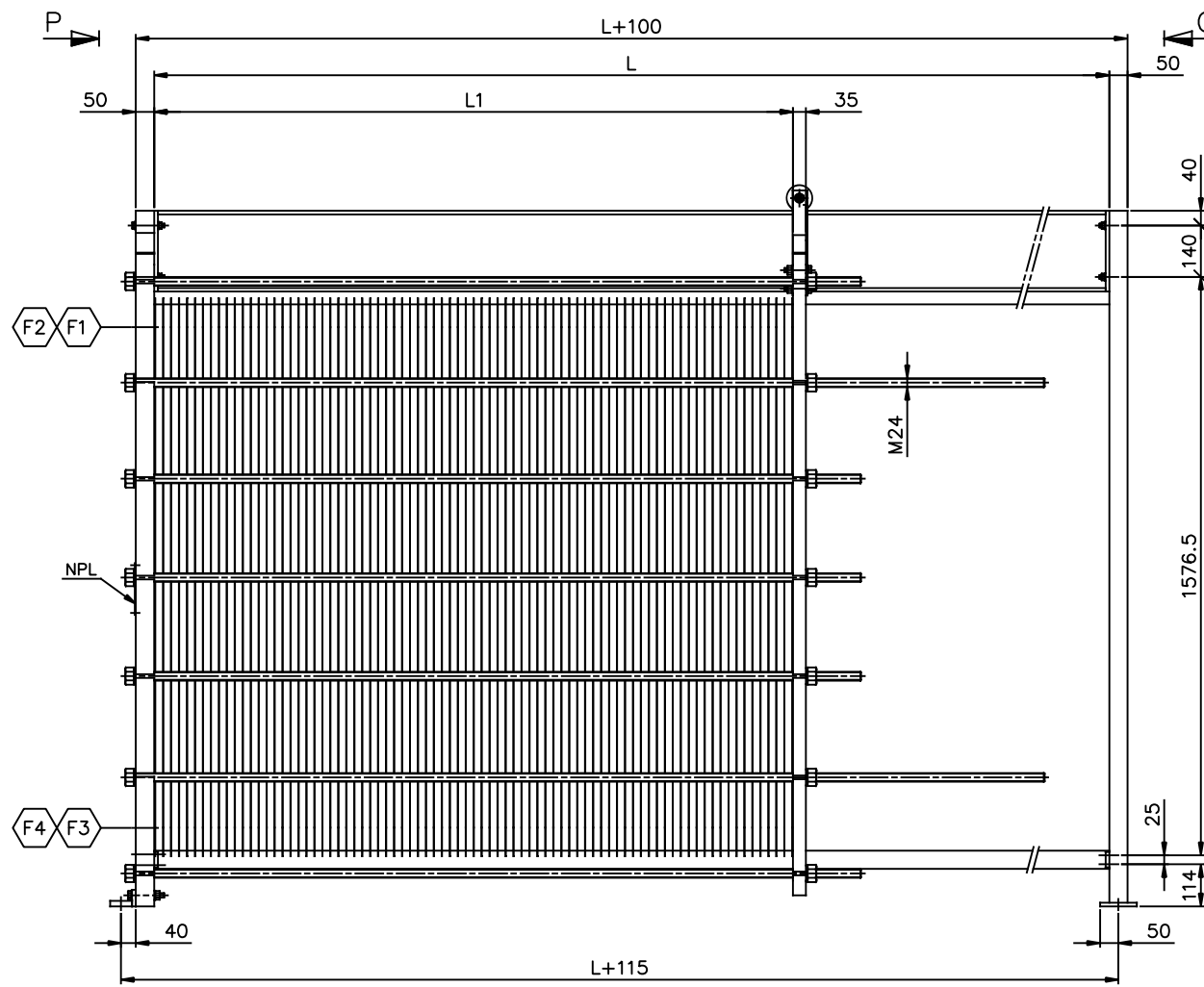
ELEVATION SCALE: 1/10
