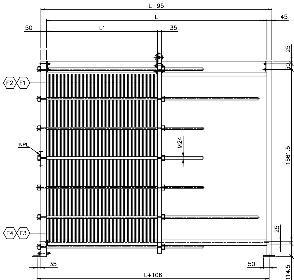
ELEVATION SCALE: 1/10
