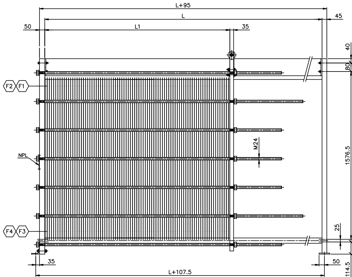
ELEVATION SCALE: 1/10
