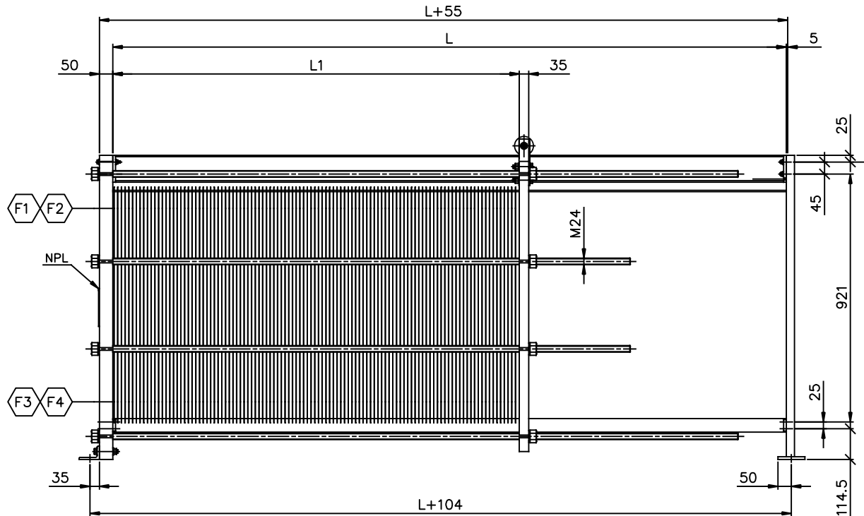
ELEVATION SCALE: 1/10
