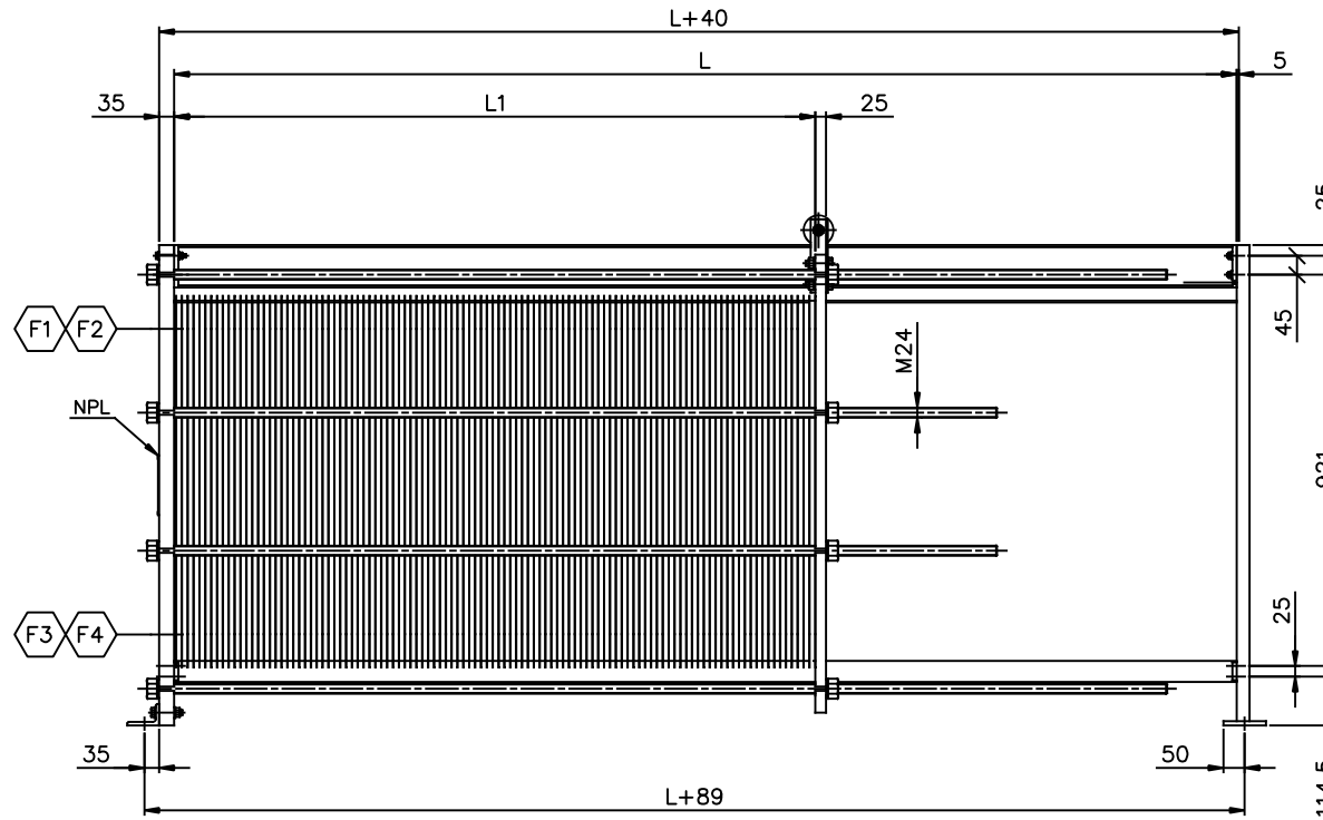
ELEVATION SCALE: 1/10
