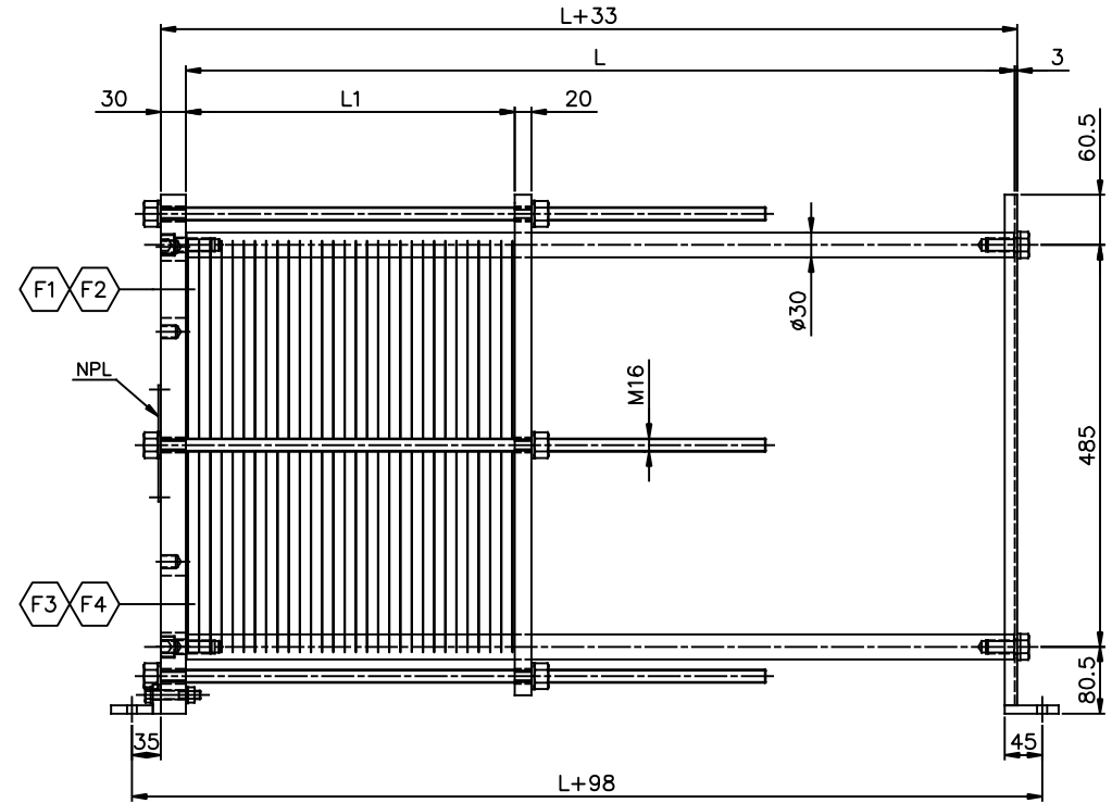
ELEVATION SCALE: 1/5
