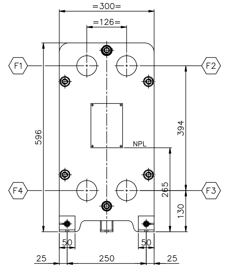
VIEW P SCALE: 1/5
