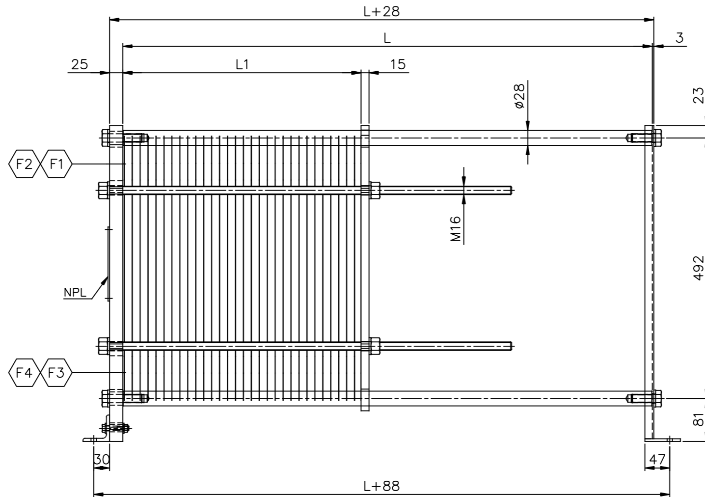
ELEVATION SCALE: 1/5
