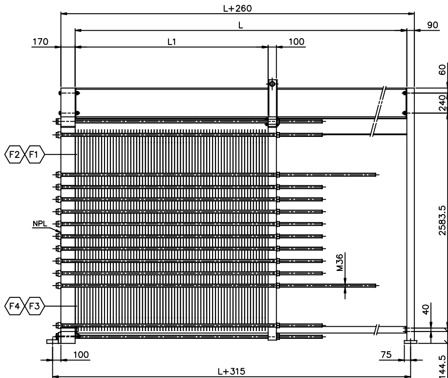
ELEVATION SCALE: 1/20
