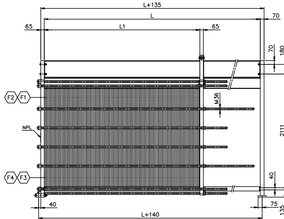
ELEVATION SCALE: 1/20
