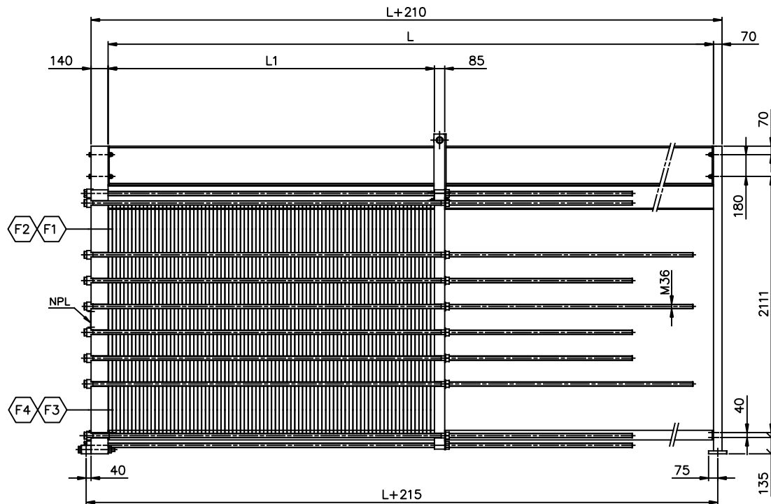
ELEVATION SCALE: 1/20
