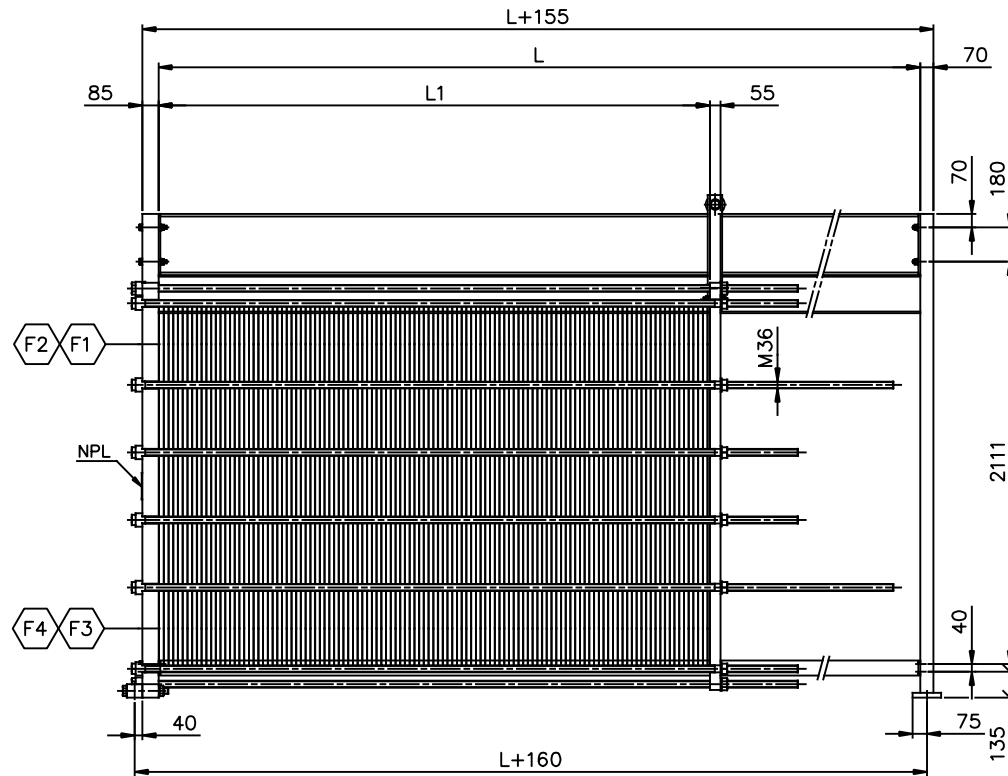
ELEVATION SCALE: 1/20
