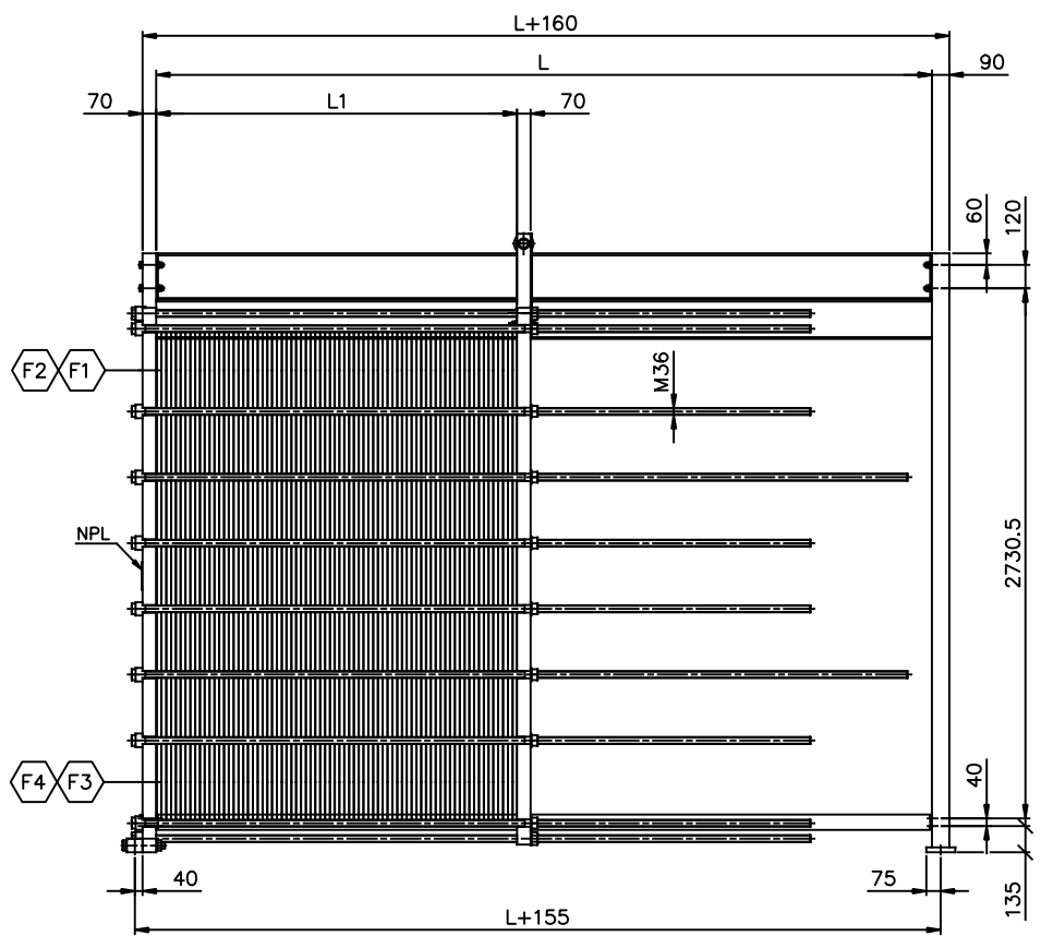
ELEVATION SCALE: 1/20
