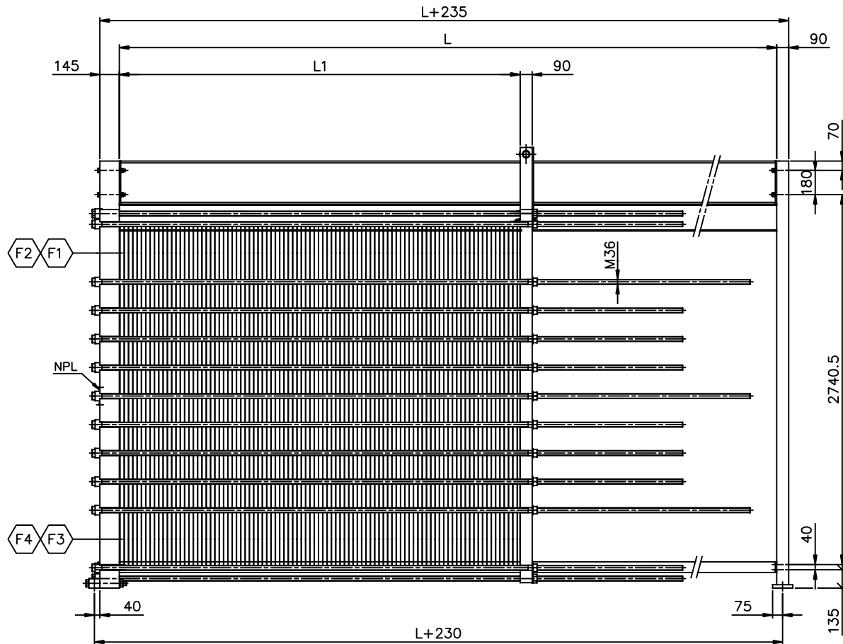
ELEVATION SCALE: 1/20
