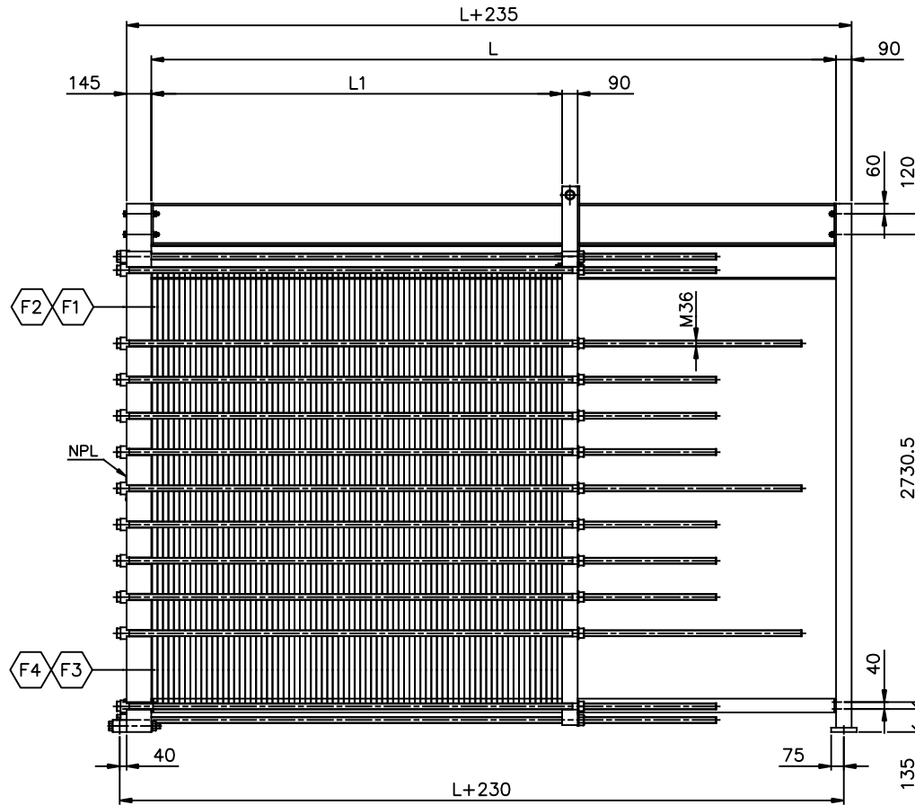
ELEVATION SCALE: 1/20
