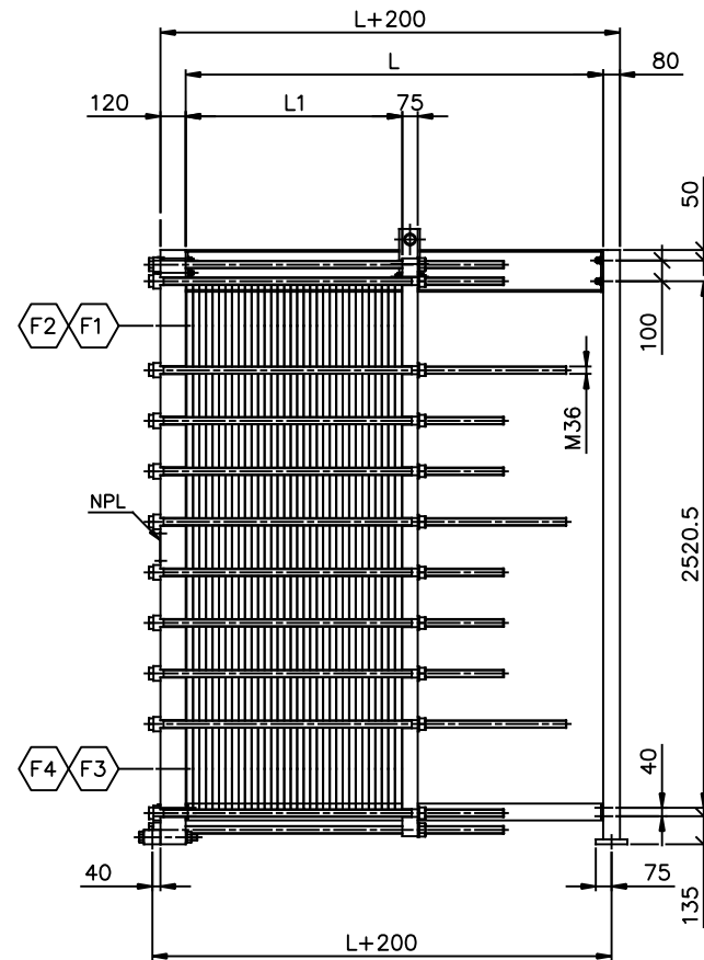
ELEVATION SCALE: 1/20
