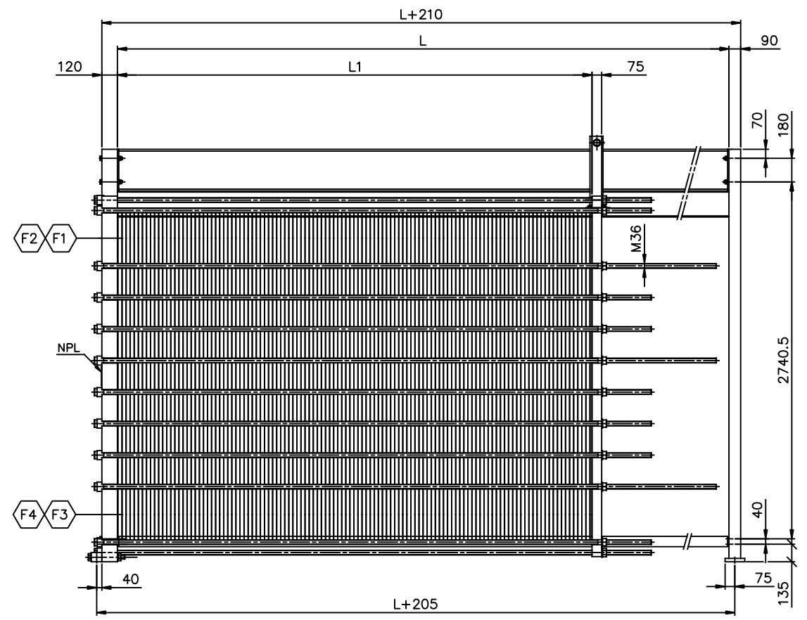
ELEVATION SCALE: 1/20
