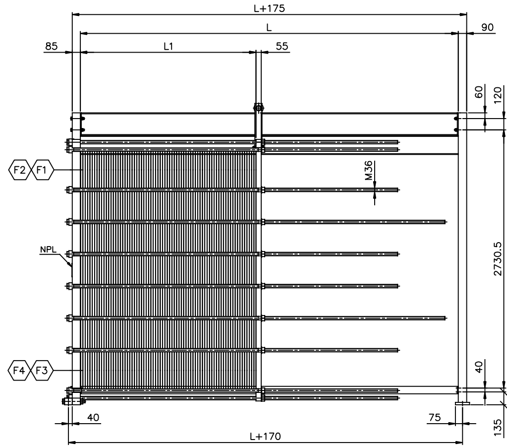
ELEVATION SCALE: 1/20
